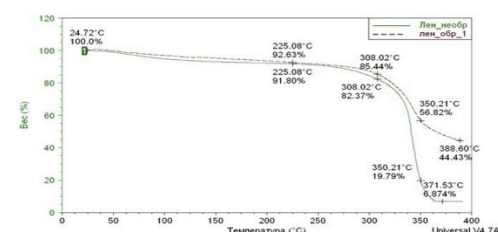
Рисунок 1 – ТГА исходного льняного волокна и обработанного борной кислотой
