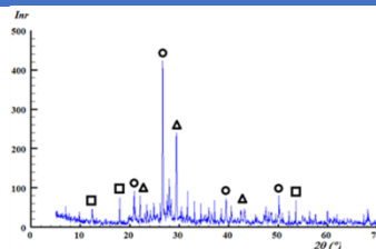
Рисунок 1 – Рентгенограмма бурового шлама Морозовского месторождения (○ – кварц; Δ – содалит; □ – каолинит)
