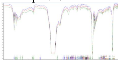
Рисунок 1 – ИК-спектры образцов ПЭ пленки: исходного (синий), модифицированного в ВЧЕ плазме аргона (красный), модифицированного в ВЧЕ плазме воздуха (зеленый)
