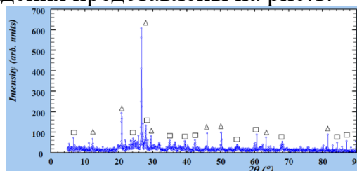
Рисунок 1 – Рентгенограмма бурового отхода Восточно-Чумаковского месторождения (Δ – кальцит, □ – кварц)
