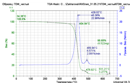
Рисунок 1 – Кривая ТГА полиэфирного волокна
