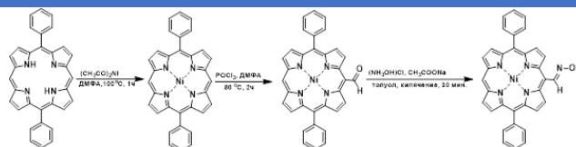
Рисунок 1 – Получение оксима мезоформил-5,15-дифенилпорфирина
