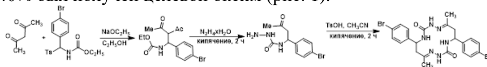
Рисунок 2 – Получение пара-бромфенил-1,2,4,8,9,11-гексаазатетрадека-7,14-диен-3,10-диона
