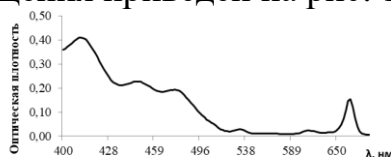
Рисунок 1 – Спектры поглощения экстракта листьев облепихи в гексане.
