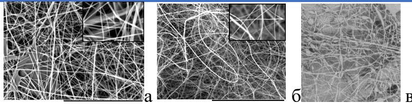
Рисунок 1 – Микрофотография волокон, полученных из смесевых композиций ПЭУ латекс : ПВС: а) состав композиции Аквапол®10:ПВС = 1:1; б) состав композиции Аквапол®10:ПВС = 4:1; в) состав композиции Аквапол®21:ПВС = 2:1. Увеличение 2000.
