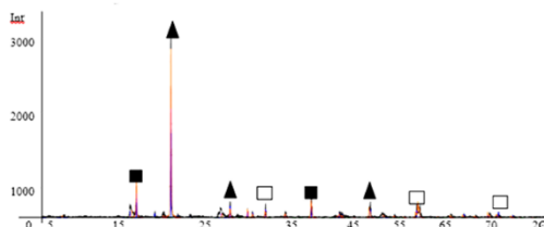
Рисунок 2 – Рентгенограмма глины Губского месторождения (▲ – кварц, ■ – монтмориллонит, □ – гидрослюда)
