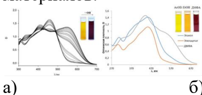
Рисунок 1 – Изменения в электронных спектрах поглощения соединения 4e: а) при различных значениях pH; б) в различных растворителях
