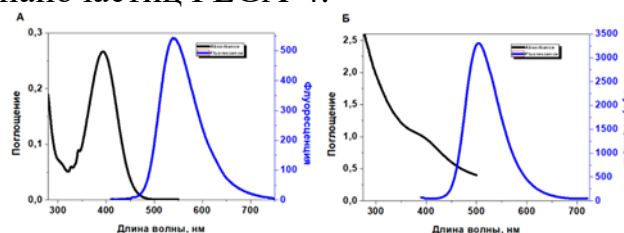
Рисунок 2: А) Спектры поглощения и флуоресценции полимера PLGA-4 в ДМСО, концентрация PLGA-4 – 12,0 мг/мл; Б) Спектры поглощения и флуоресценции наночастиц PLGA-4 в воде, концентрация 2,5 мг/мл
