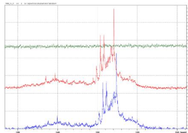
Рисунок 1 – Диапазон от 120 до 150 13С ЯМР спектров исследованных образцов. Зелёным цветом обозначен спектр детского масла, красным – косметического вазелина, синим – индустриального масла.
